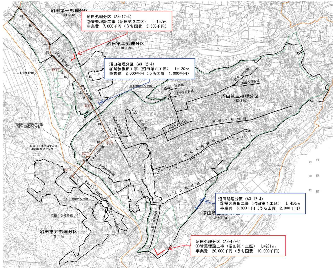
沼田市(A1-1)(沼田処理分区)計画図
