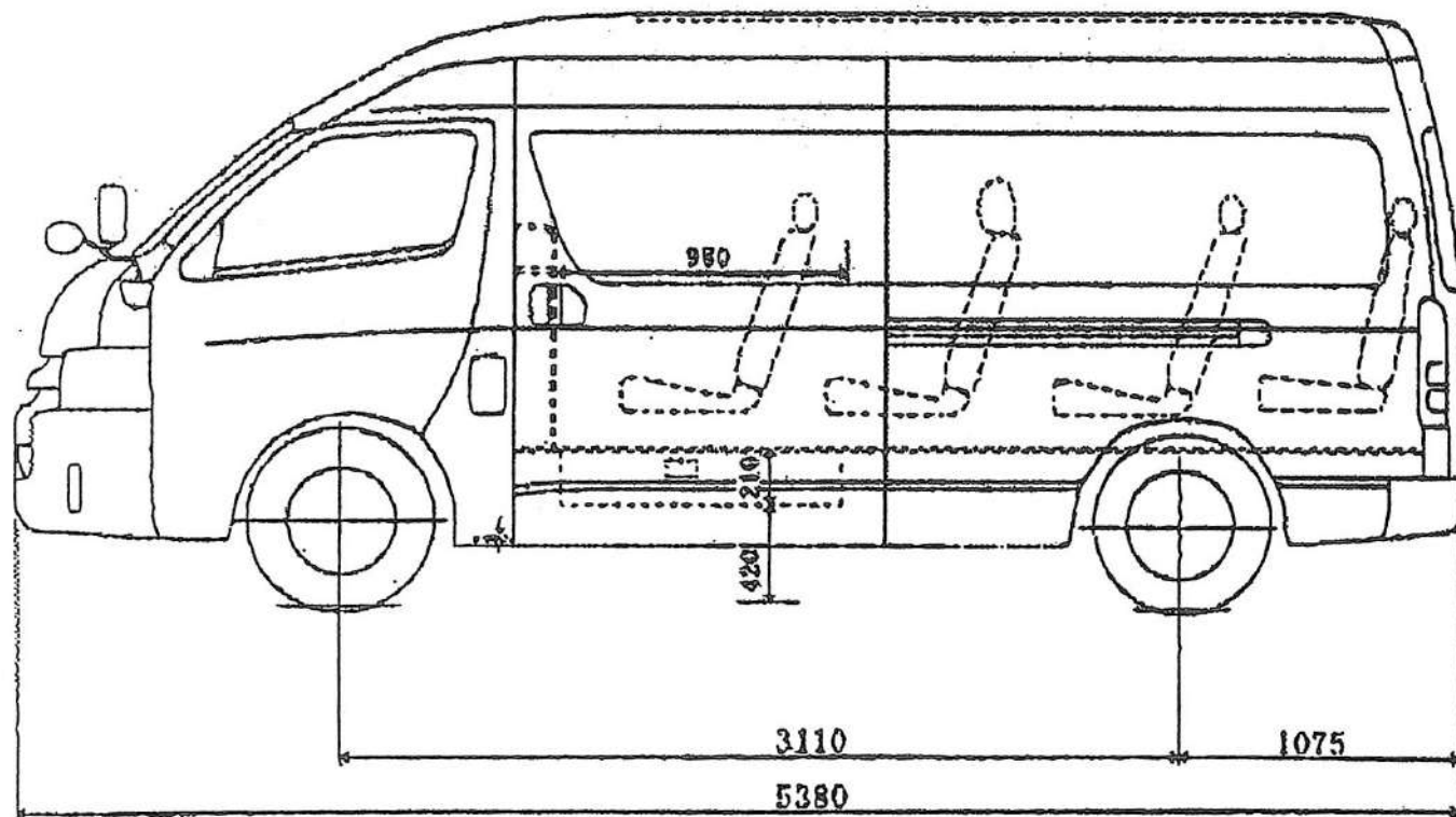
トヨタ自動車製 ワゴン車 ハイエース コミューターサイズ 14人乗り（運転手1名 乗客13名）
